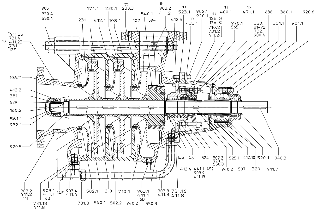
Рисунок 52: Multitec - тип компоновки А - типоразмер 125-150
