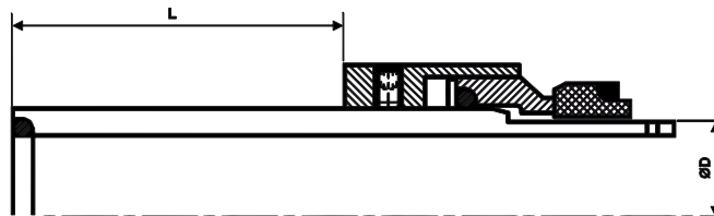
Рисунок 42: Установочный размер L для торцевого уплотнения
