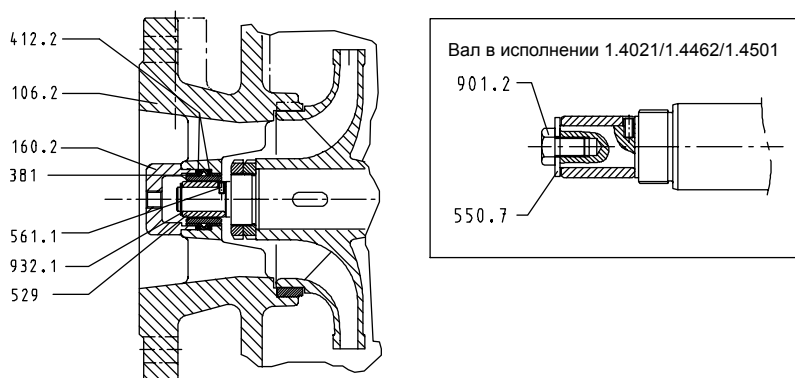
Рисунок 21: Демонтаж подшипников скольжения - аксиальный всасывающий патрубков
