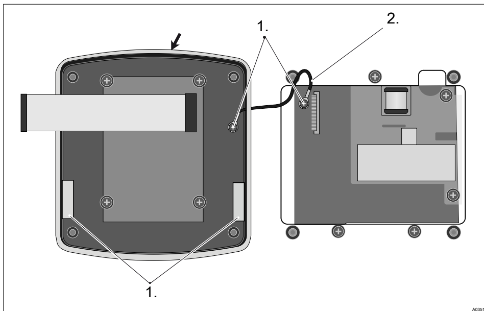
Рис. 9: Установка профильного уплотнения на верхней части корпуса регулятора
