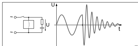
Рис. 15: Процесс отключения на осциллограмме
