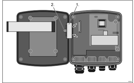
Рис. 53: Демонтаж шарнира
