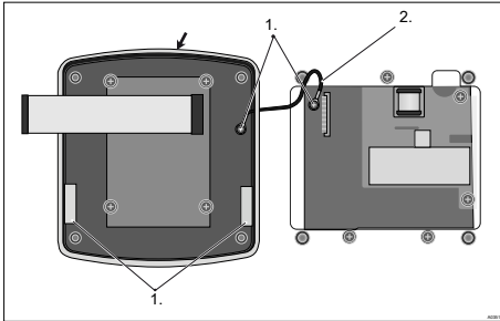
Рис. 57: Установка профильного уплотнения на верхней части корпуса регулятора
