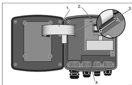
Рис. 47: Снятие плоского кабеля
