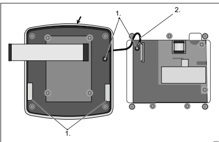
Рис. 44: При встройке в распределительный щит: Установка профильного уплотнения на верхней части корпуса регулятора
