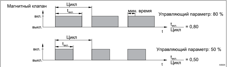
Рис. 39: Электромагнитный клапан (= P-REL: dosing)
