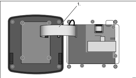
Рис. 52: Отсоединение плоского кабеля от корпуса
