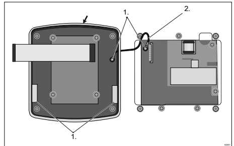
Рис. 54: Демонтаж ленты для снятия нагрузки
