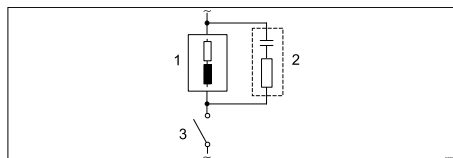
Рис. 16: RC-блок схемной защиты для контактов реле
