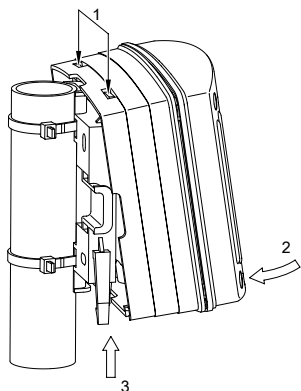
Рис. 4: Подвесьте и закрепите регулятор DULCOMETER® Compact
