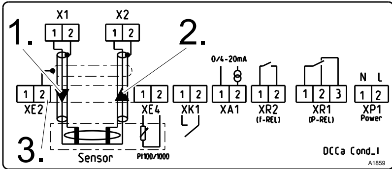
Рис. 11: Наклейка со схемой расположения клемм регулятора Compact
