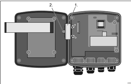
Рис. 43: Демонтаж шарнира
