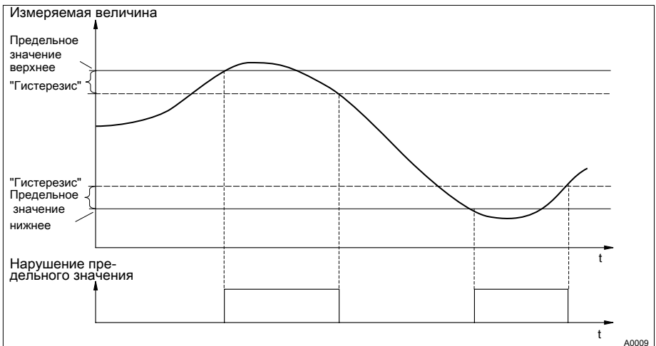
Рис. 38: Гистерезис
