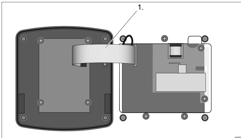
Рис. 10: Вставьте плоский кабель в цоколь и зафиксируйте его
