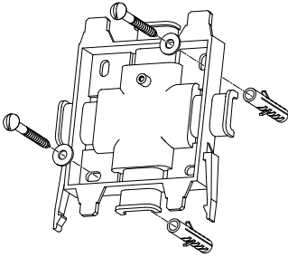
Рис. 2: Привинтите крепление для стены/трубы с использованием подкладных шайб
