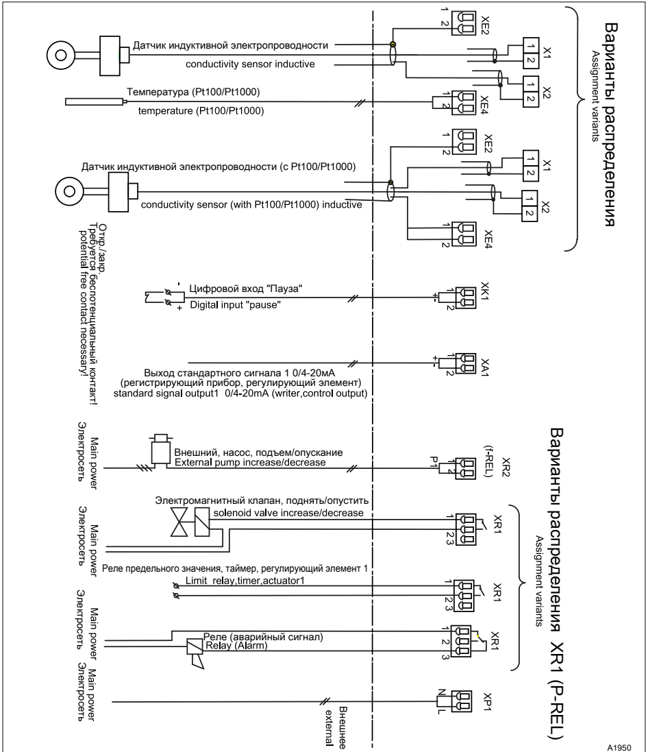
Рис. 13: Схема клеммных соединений
