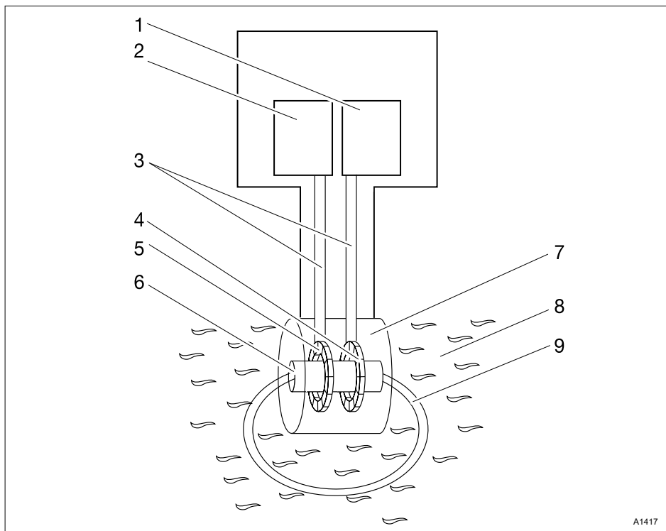
Рис. 17: Принцип измерения
