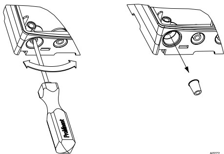
Рис. 14: Выламывание резьбовых отверстий
