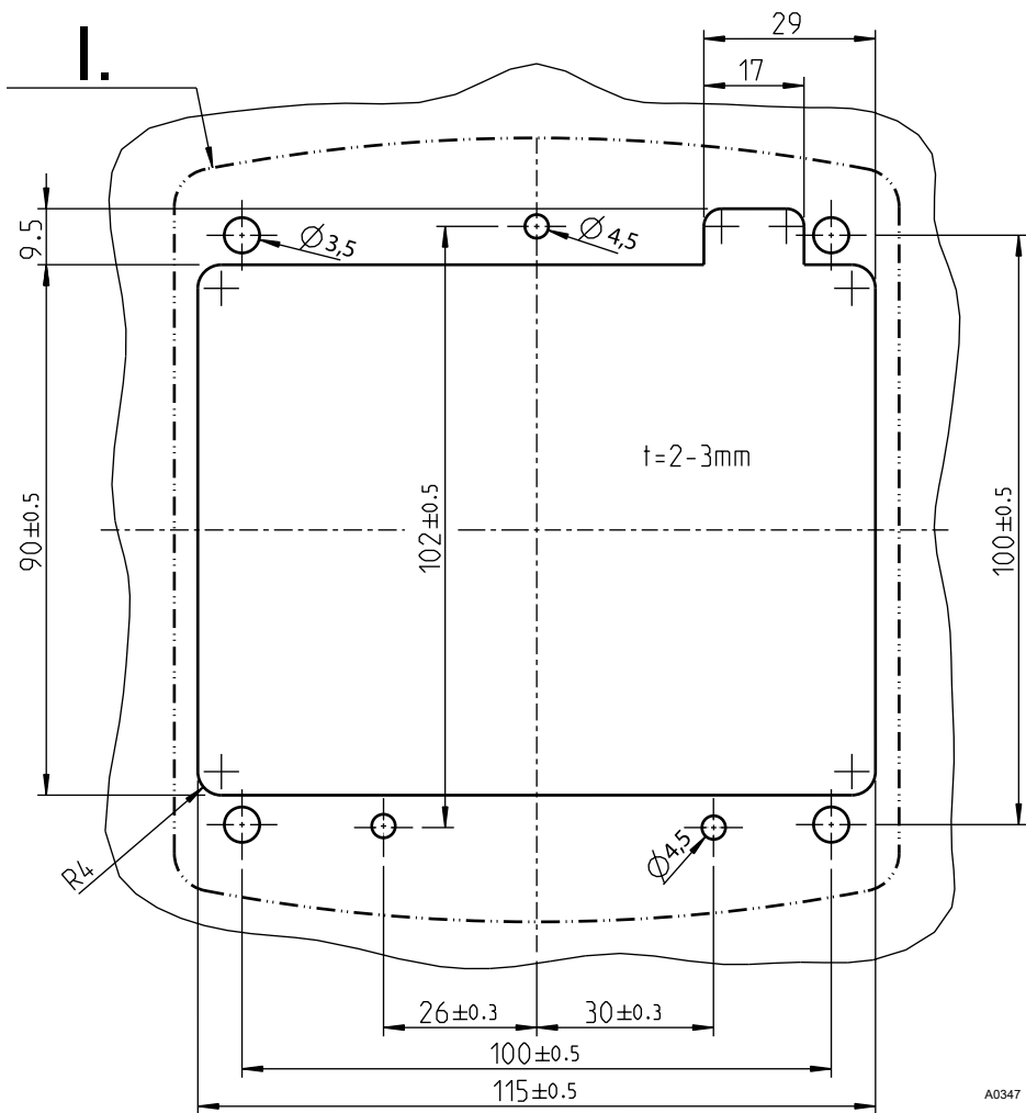
Рис. 5: Чертеж не соответствует масштабу и служит исключительно для информации.
