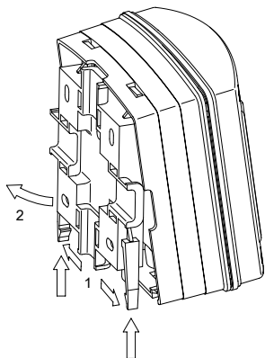
Рис. 46: Демонтаж крепления для стены/трубы
