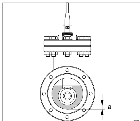
Рис. 32: Расстояние до стенки [a]
