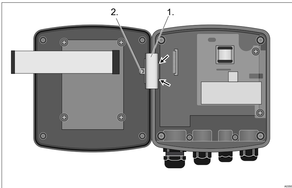
Рис. 7: Демонтаж шарнира
