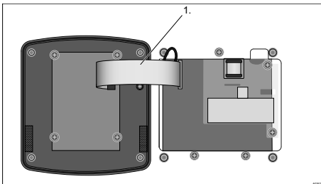
Рис. 58: Вставьте плоский кабель в цоколь и зафиксируйте его
