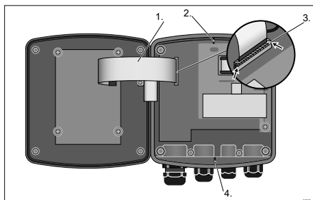
Рис. 50: Закрепите плоский кабель
