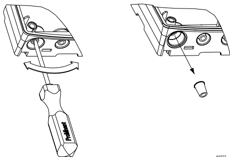
Рис. 55: Выламывание резьбовых отверстий
