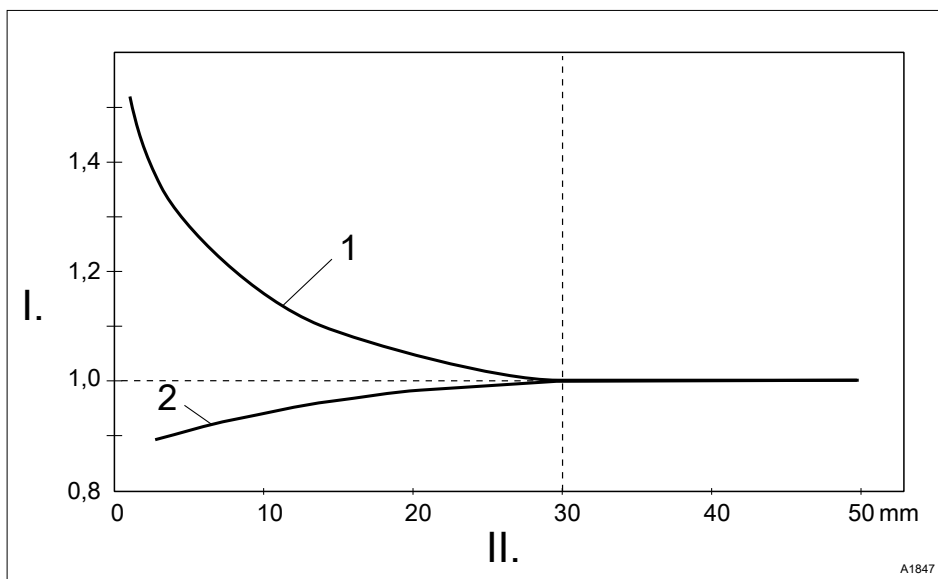
Рис. 31: Зависимость монтажного коэффициента от расстояния до стенки
