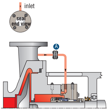
A - orifice
