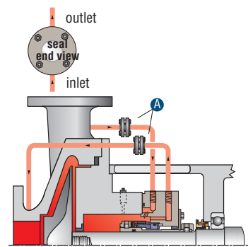
A - orifice
