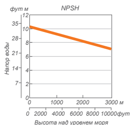
Атмосферное давление в напоре воды на различных высотах.
