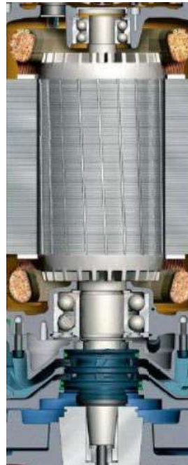
Вал и подшипники насоса
