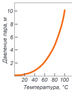
Давление пара для воды при различных температурах
