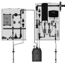
P_PMA_BEZ_0096_SW CDKc 420 (на изображении показано опциональное оснащение)
