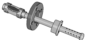
pk_7_011_2 Погружная труба от DN 100
